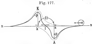
Schema für den In- und Dekrementsatz. [Gleichzeitig Superposition der positiven und negativen Polarisationskurve (nach Hermann)].
